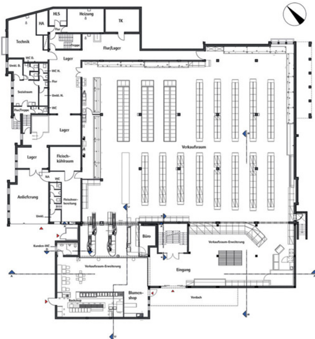
Grundriss Untergeschoss
