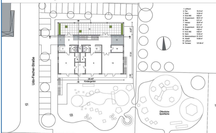
Grundriss Obergeschoss
