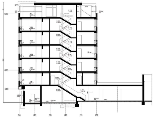
Schnitt B-B
