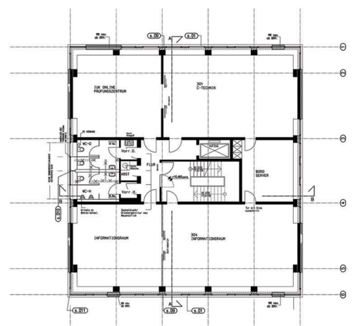
Grundriss 3. Obergeschoss
