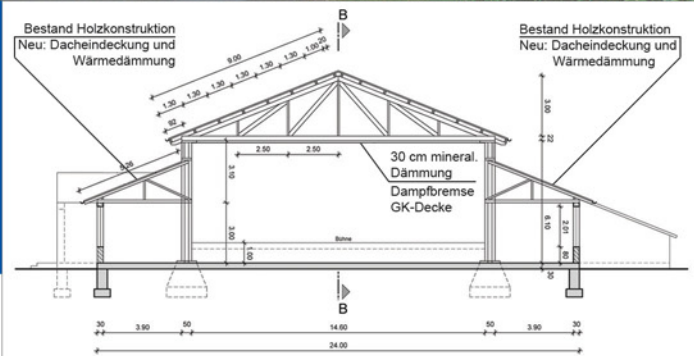
Schnitt A-A
