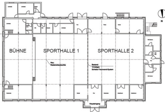
Grundriss Erdgeschoss
