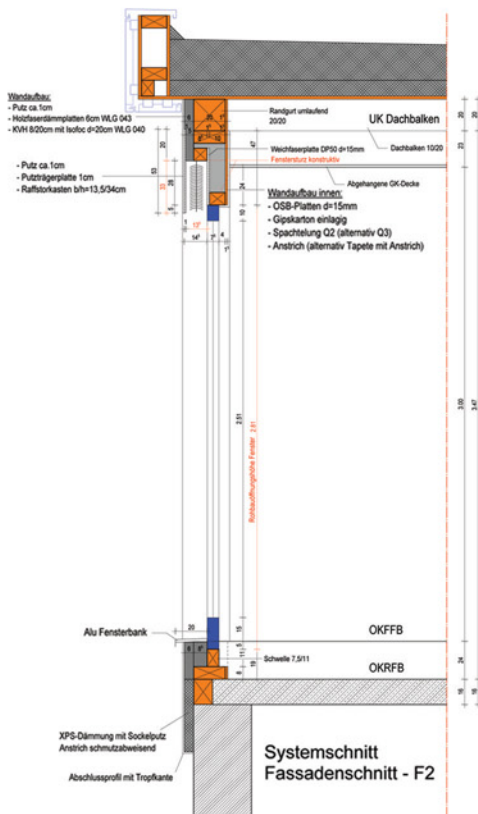
Fassadenschnitt
