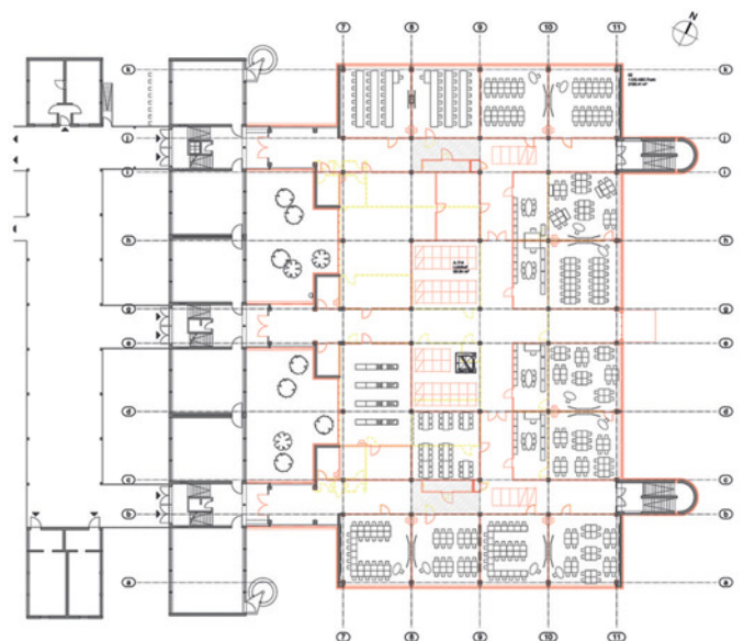
Grundriss 1. Obergeschoss - Werkplanung
