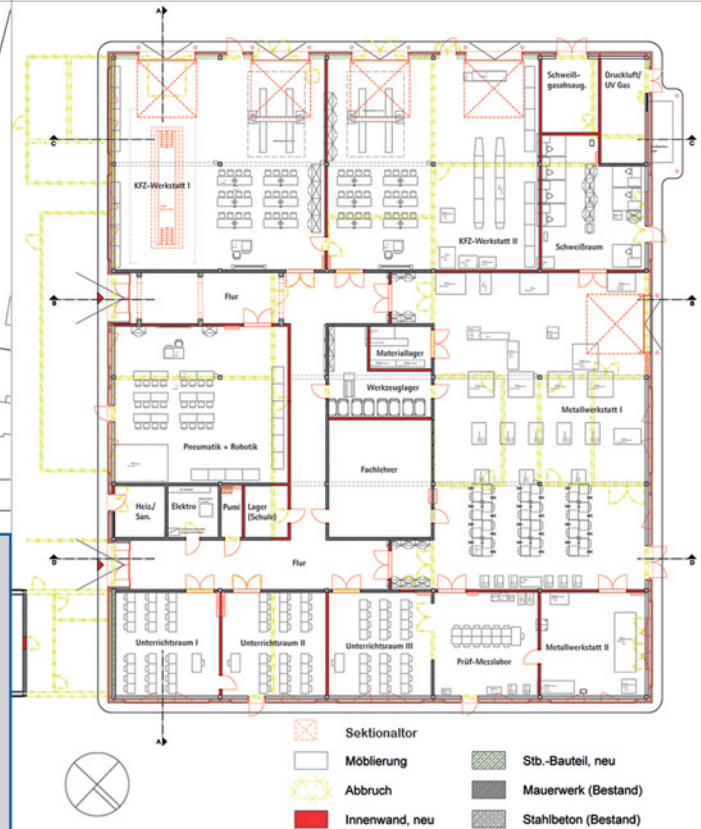
Grundriss Erdgeschoss Werkhalle
