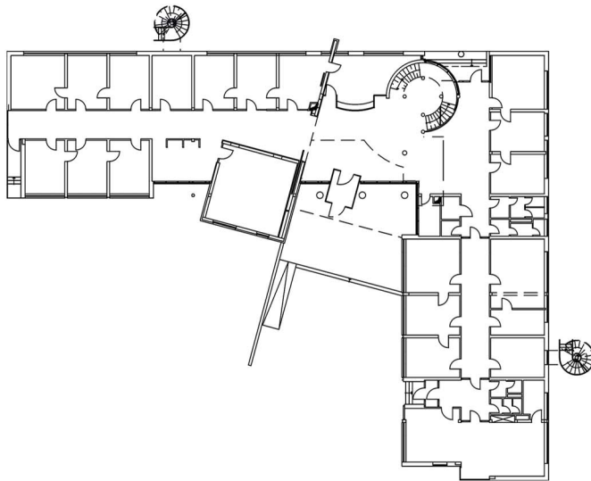
Grundriss Erdgeschoss
