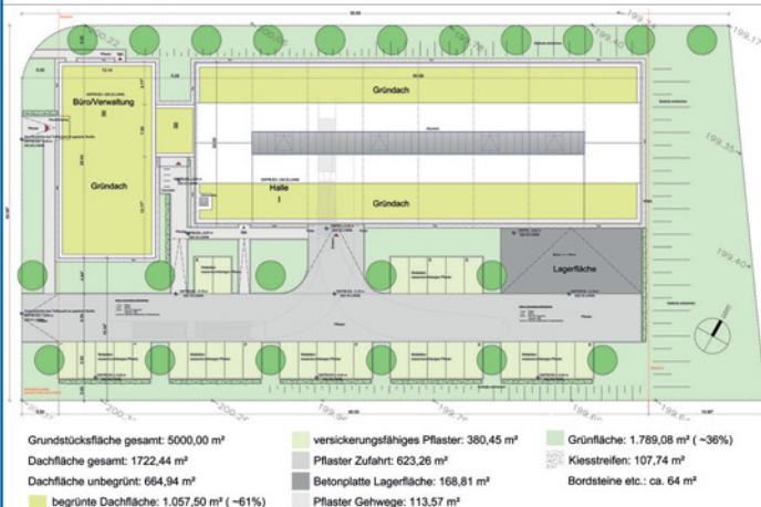
Freiflächenplan
