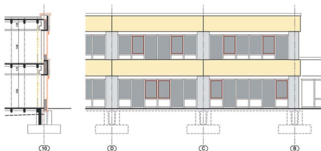
Fassadenkonzept
